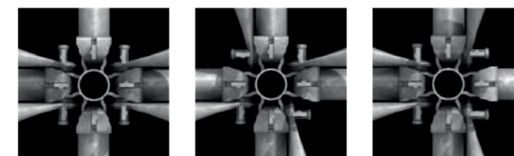
▲ Le nœud CRAB permet la fixation simultanée de 8 éléments : 4 moises et 4 diagonales.
